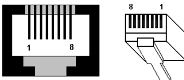
Rys. Widok gniazda i wtyku RJ-45 8/8
